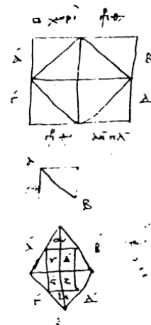
Abbildung 1. Konstruktionszeichnung zum Problem der Quadratverdoppelung in den Scholien zu Plato, Men. 82 b ff., im Cod. Vindobonensis suppl. Graec. 7 , fol. 418r (10. Jh.).
